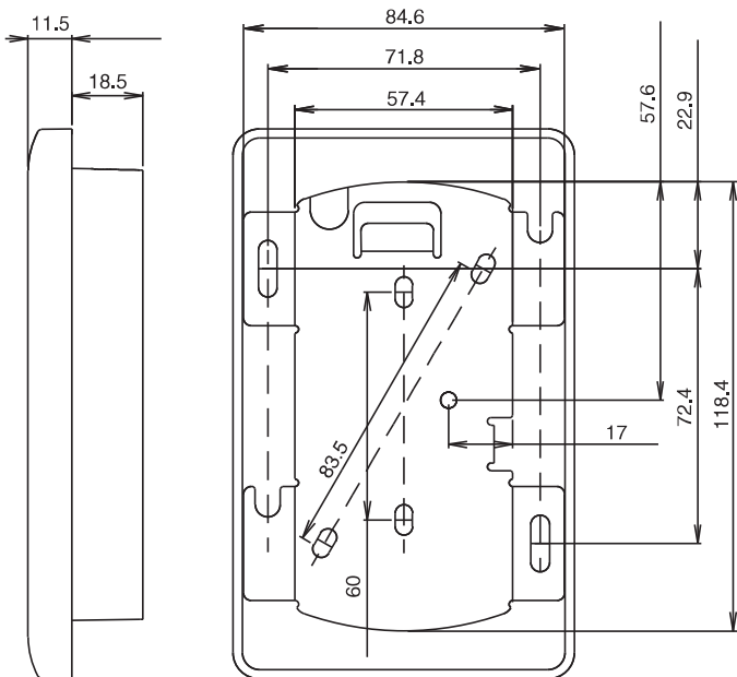
Dimensions
