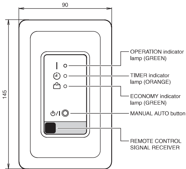
Dimensions
